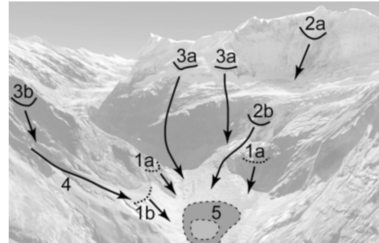
1a) Felssturz 1b) Moränenrutschungen 2b) Eislawinen Steilgletscher 3a) Permafrostdegradation 3b) Steinschlag Mättenberg 4) Murgangaktivität mit Erosion auf Seitenmoräne 5) Gletschersee. Quelle: Haerberli et al. 2010
